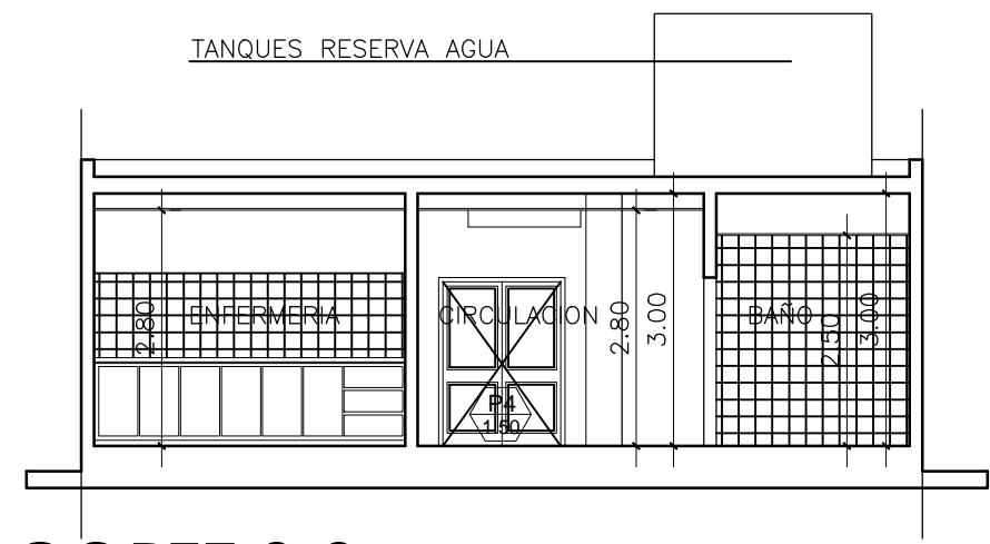
CORTE 2-2
