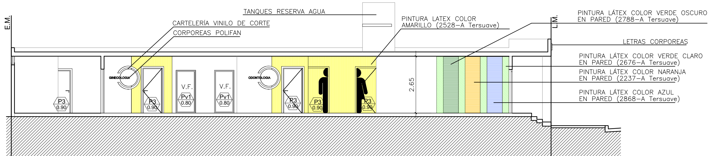
FACHADA
